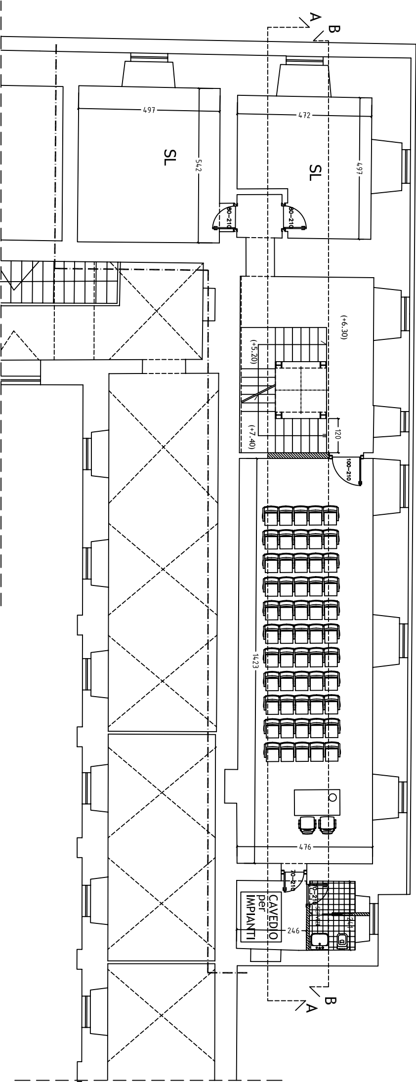
PIANTA PRIMO PIANO - quota (+6.30m)
